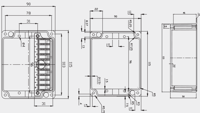
Dimension (Allowable error:± 1mm)
