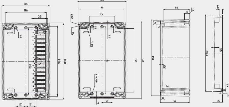
Dimension (Allowable error:± 1mm)
