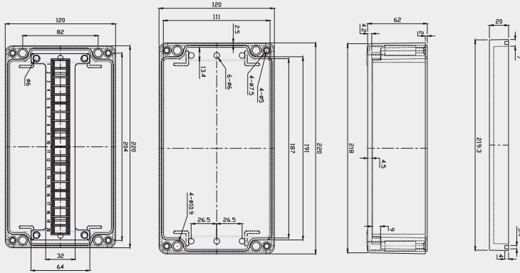
Dimension (Allowable error:± 1mm)
