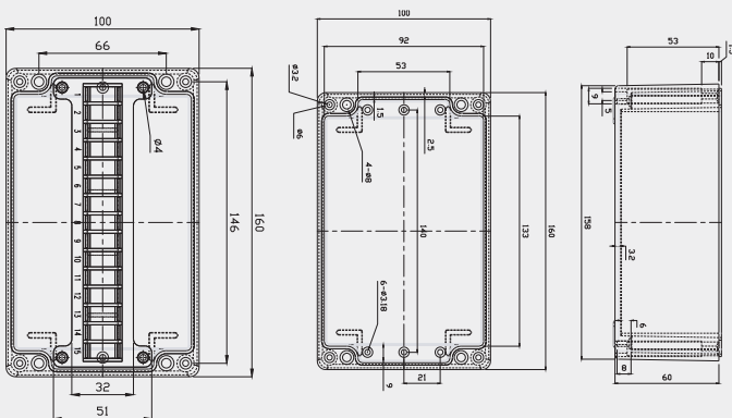
Dimension (Allowable error:± 1mm)
