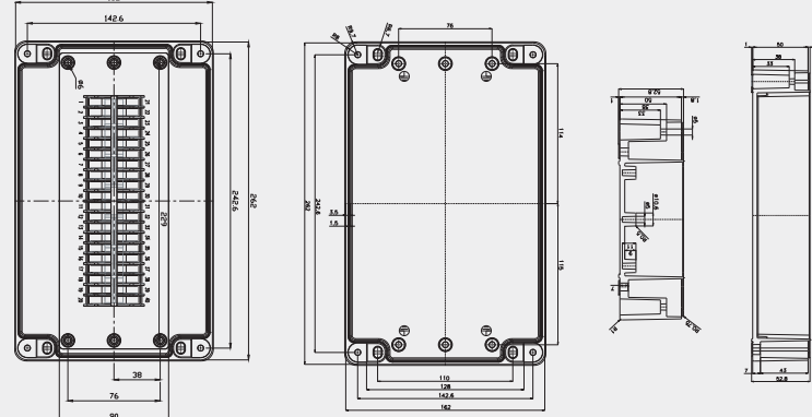
Dimension (Allowable error:± 1mm)
